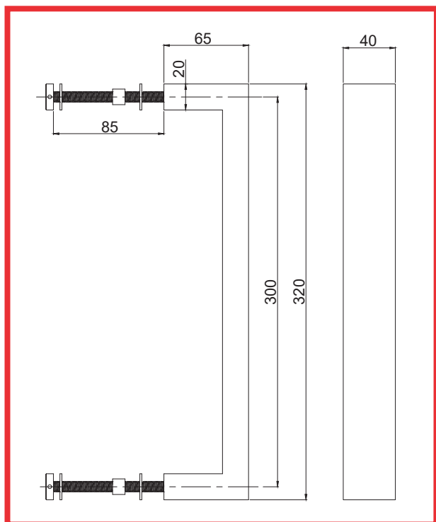
Esquema lineal
