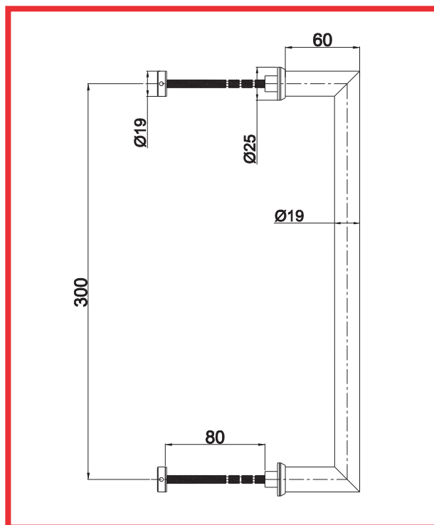
Esquema lineal
